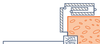
Ferrage sur montants cornière 1 vantail en tableau, les autres en façade
