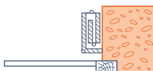
Pose sur tapées incorporées bois ou pvc
