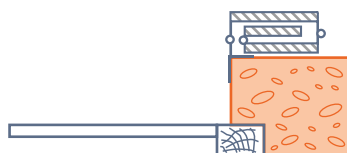
Ferrage sur montants cornière emboîtant l'angle du tableau
