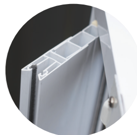
Détail joint et battement
