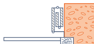
Pose sur tapées aluminium
